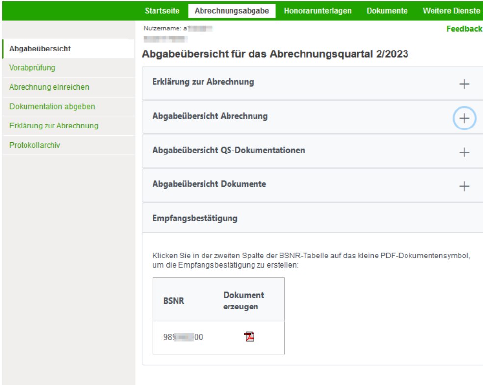
Abbildung 33: Abgabeübersicht
