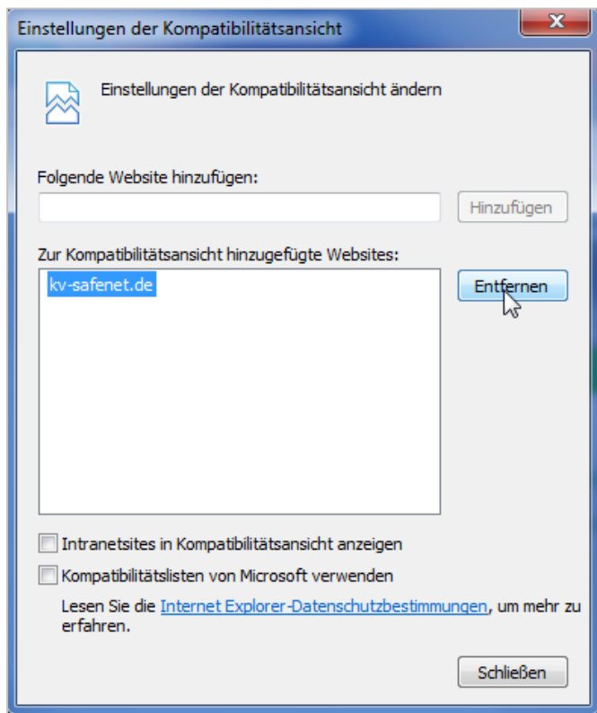
Abbildung 1: Kompatibilitätsansicht entfernen
