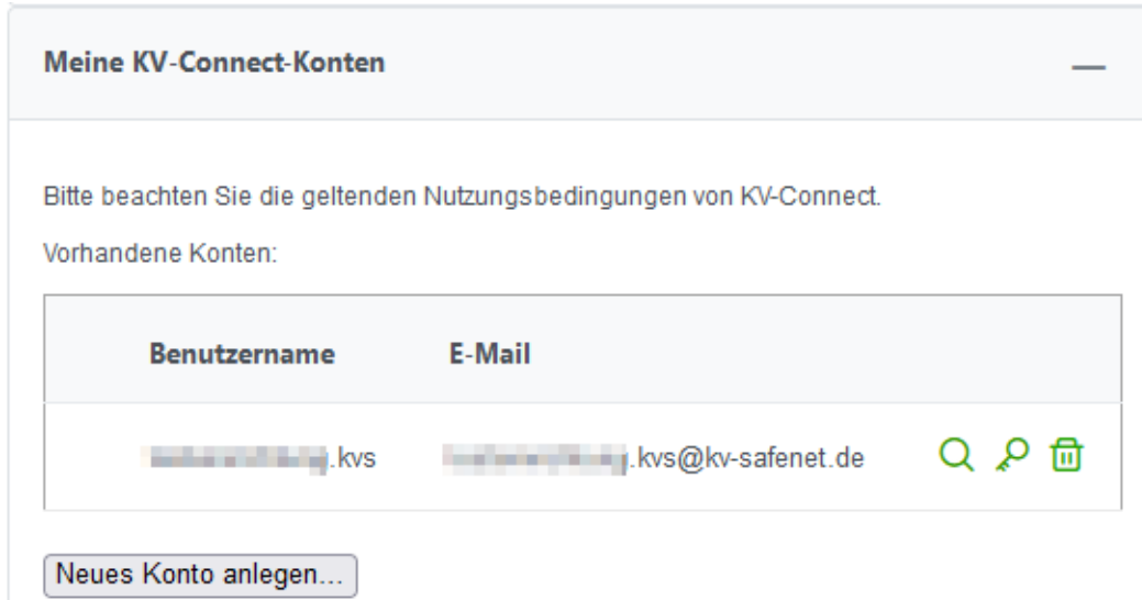
Abbildung 22: Kontoübersicht
