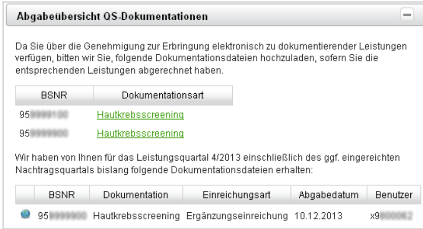
Abbildung 35: Abgabeübersicht Qualitätssicherungs-Dokumentationen
