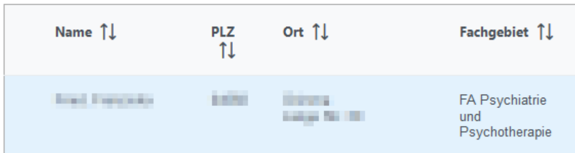
Abbildung 30: Hinweismeldung Fachgebiete
