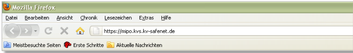
Abbildung 2: Aufruf
