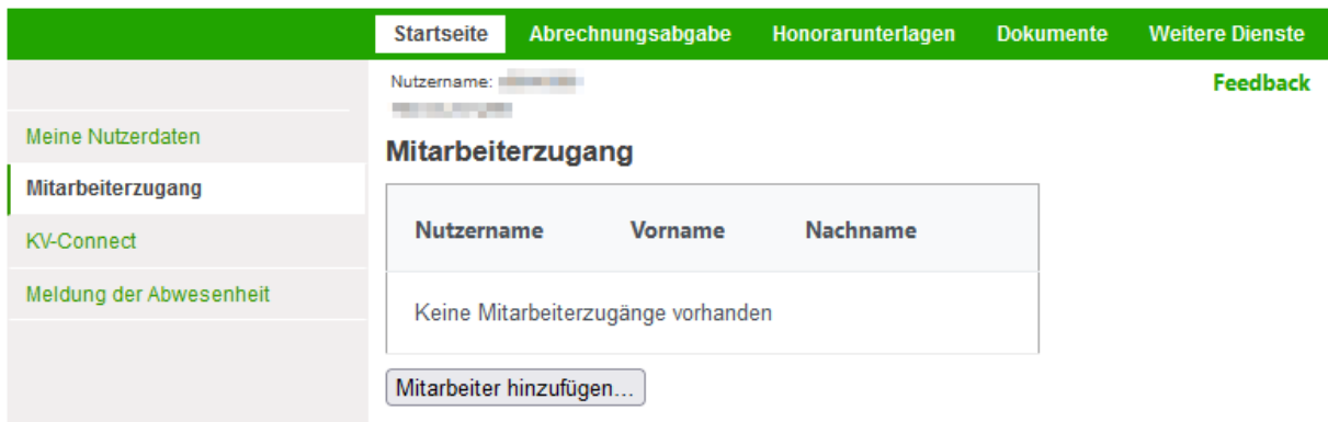
Abbildung 9: Navigation Mitarbeiterzugang
