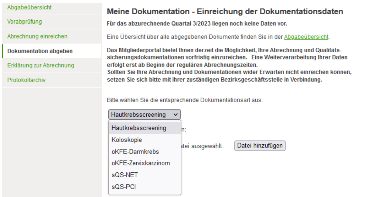
Abbildung 52: Dokumentation abgeben
