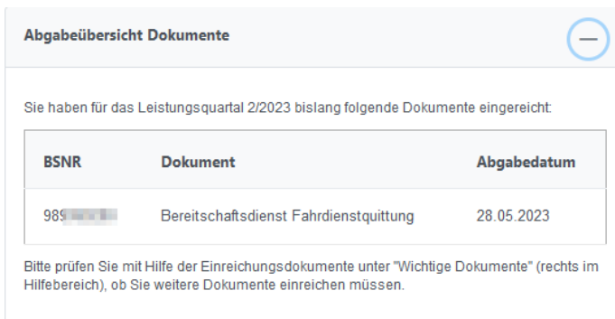
Abbildung 36: Abgabeübersicht Dokumente
